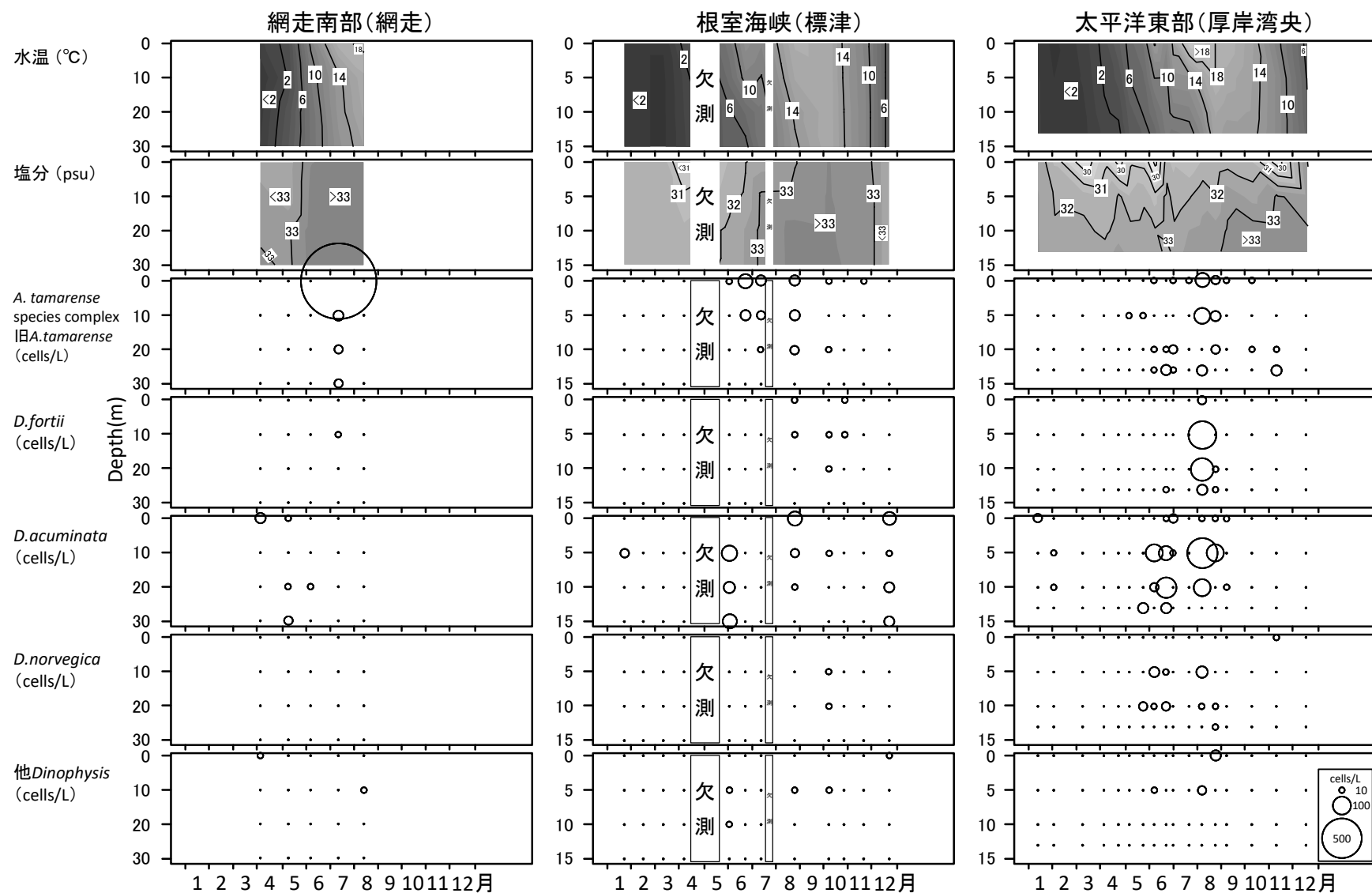
図6 網走南部(網走), 根室海峡(標津), 太平洋東部(厚岸湾中央)海域における水温・塩分と旧 A. tamarensis および Dinophysis 属の鉛直分布の季節変化
