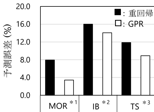
図2 実験値から算出した下限値(信頼水準75%における95%下側許容限界値)に対する重回帰およびGPR-basedモデルから算出した下限値(5パーセンタイル値)の予測誤差(*1:曲げ強度, *2:剥離強度, *3:吸水厚さ膨張率)
