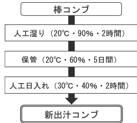
図6 新たな出汁コンブの製造工程例
