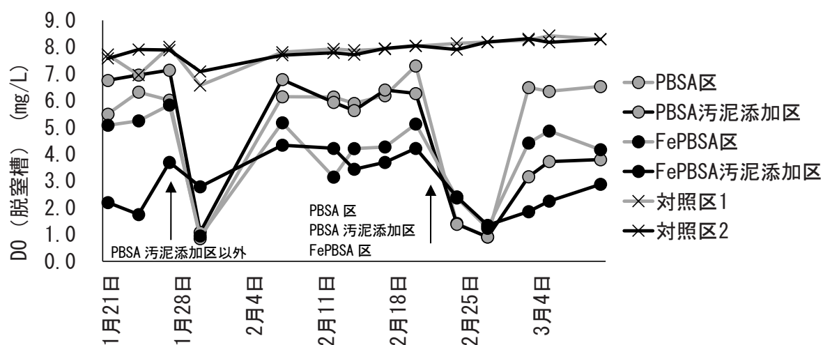
図3 脱窒槽のDOの推移 (矢印は通水を停止した日と区)
