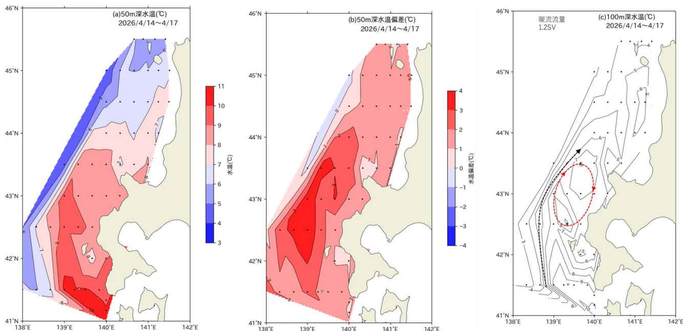
図 2026年4月中旬における (a) 50m深水温 (b) 50m深水温偏差の水平分布、(c) 100m深水温の水平分布と対馬暖流の流路（矢印）。水温偏差は過去30年（1989年～2018年）の平均値から算出。流量の単位はSv（= 1 \times 10^6 m 3 /s）。
