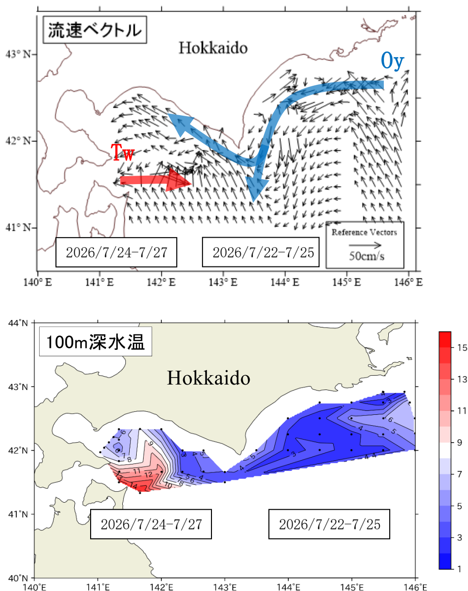
図 (上) 流速ベクトル (下) 100m深水温の水平分布
