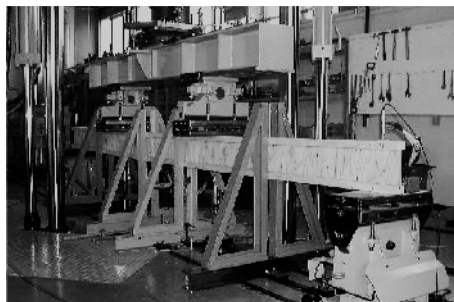
写真1 曲げ試験
