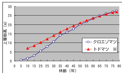
図 1 樹高成長
