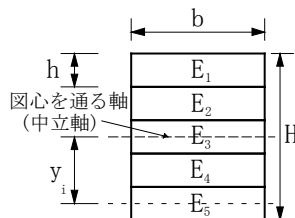
図1 5層構成の積層材料
