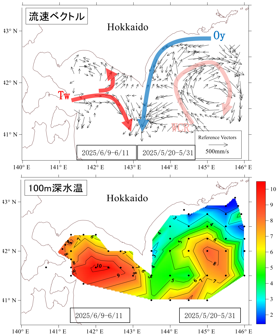
図 (上) 流速ベクトル (下) 100m深水温の水平分布
