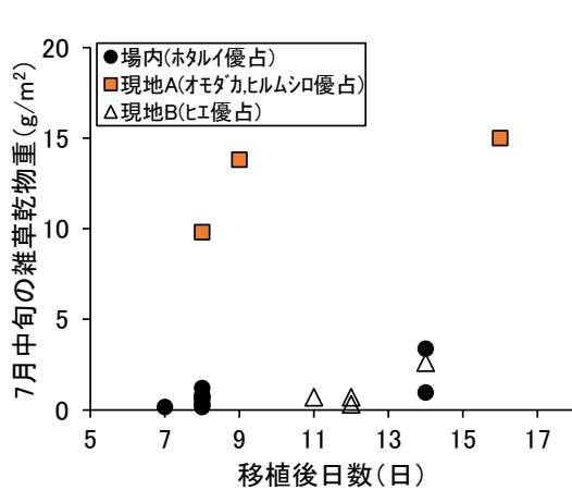
図1 1回目の機械除草時期と残草量の関係 (2020-2022年)
